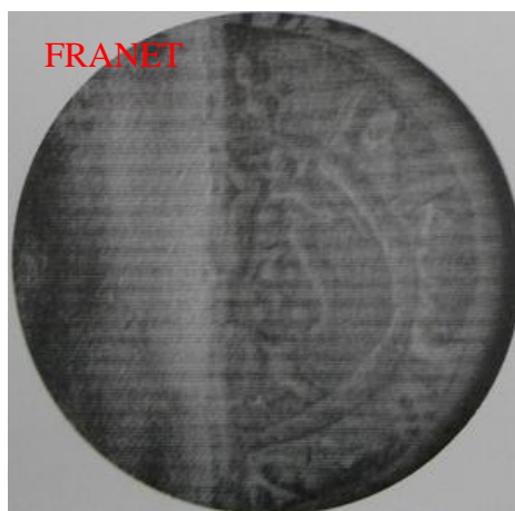
6. Banknot 20 zł – medalion – obraz w świetle białym/z lewej/ i podczerwonym
